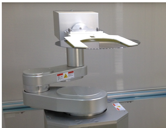
(ウエハを保持したまま 180°回転した状態)
